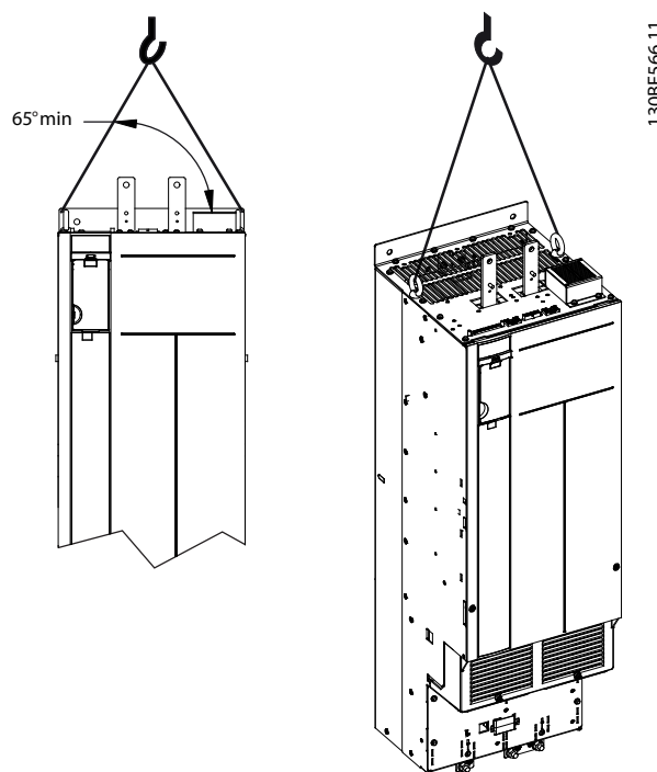
Ilustração 4.3 Içamento do conversor
