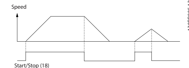
Ilustração 8.1 Partida/parada com Safe Torque Off
