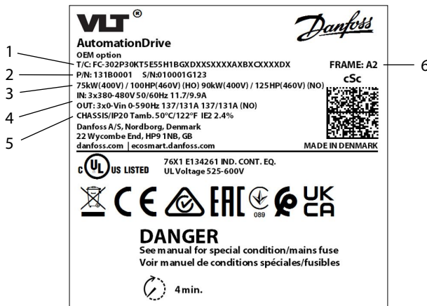
Рисунок 1: Пример паспортной таблички
