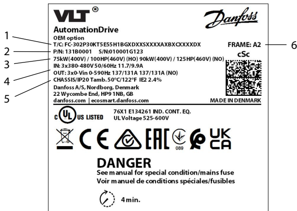
图解 1: 铭牌示例
