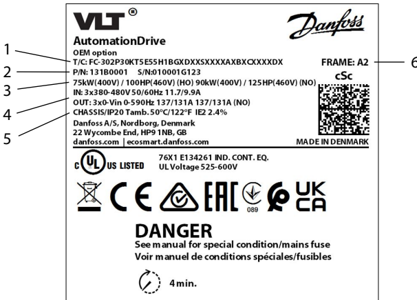
Ilustración 1: Ejemplo de la placa de características
