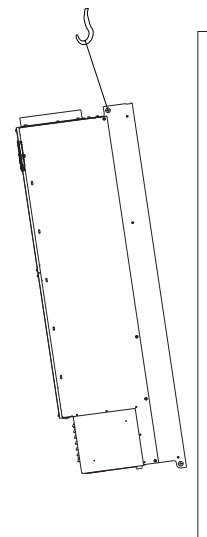
Ilustração 9.1 Método de Elevação Recomendado
