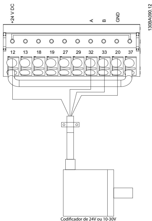
Ilustração 12.7 Configuração dos fios para o encoder
