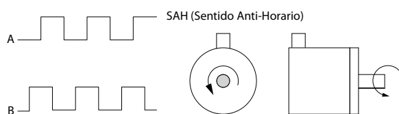
Ilustração 12.6 Determinação da direção do encoder
