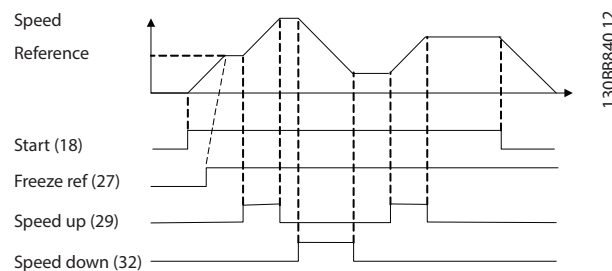
Ilustração 12.4 Aceleração/desaceleração
