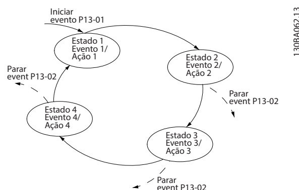
Ilustração 5.4 Ordem de execução quando 4 eventos/ações são programados
