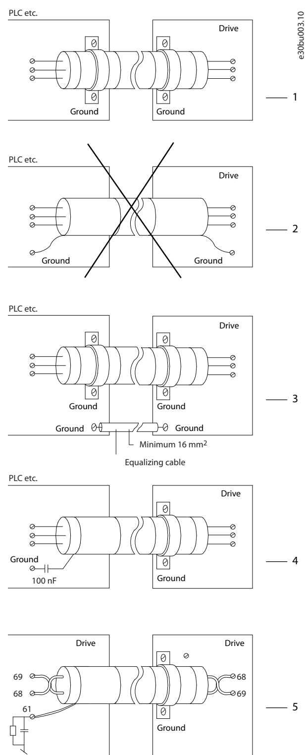
Ilustração 10.4 Exemplos de aterramento
