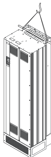
Ilustração 9.1 Método de Elevação Recomendado
