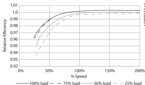
Ilustração 10.16 Curvas de eficiência típica
