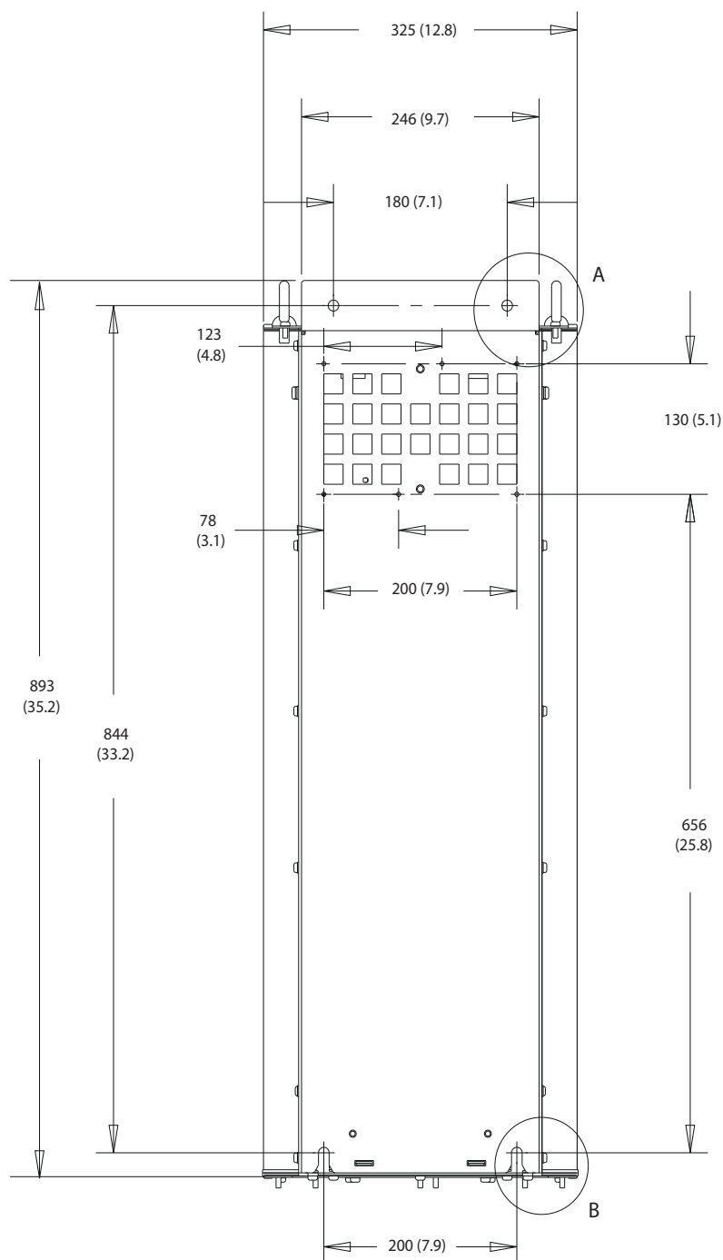
Ilustração 8.3 Vista traseira do D1h
